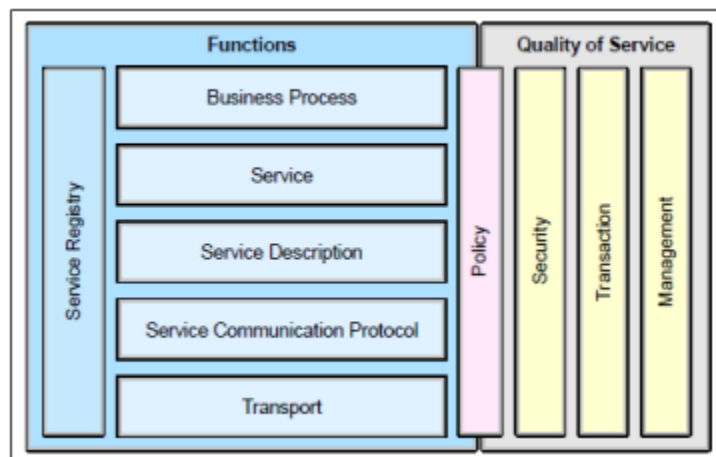
Figura 3 - SOA. Adaptado de Endrei et al. (2004)
